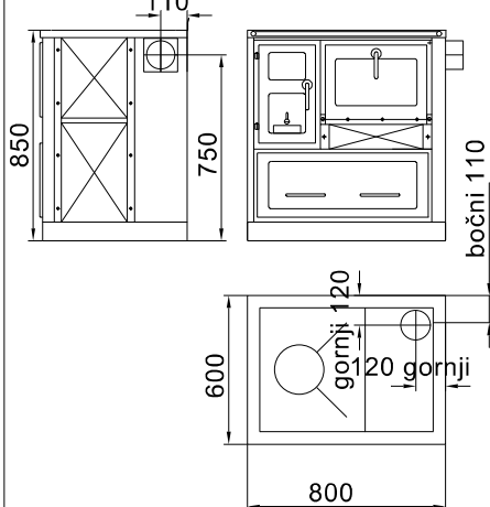
VILMA 8kW s pečnicom
