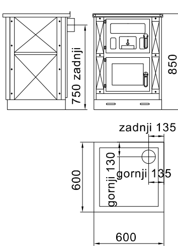
LJUBICA CENTRAL 24kW s pečnicom
