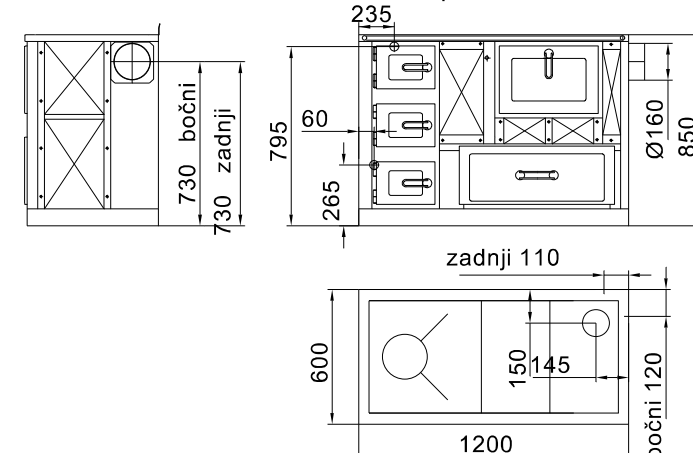
ŠTEFANIJA CENTRAL 38kW
