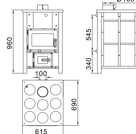
ŠTEFANIJA CENTRAL 38kW
