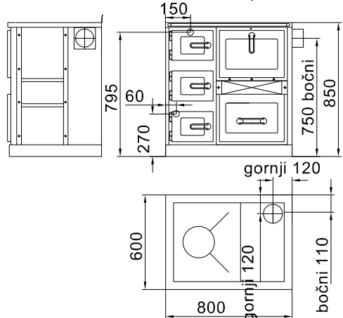
GITA CENTRAL 24kW bez pečnice
