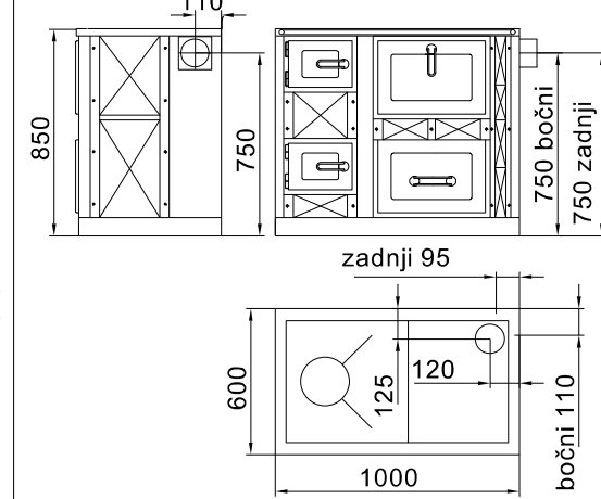
JASMINA 10kW s pečnicom
