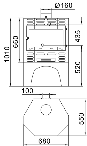
VILMA CENTRAL 20kW s pečnicom
