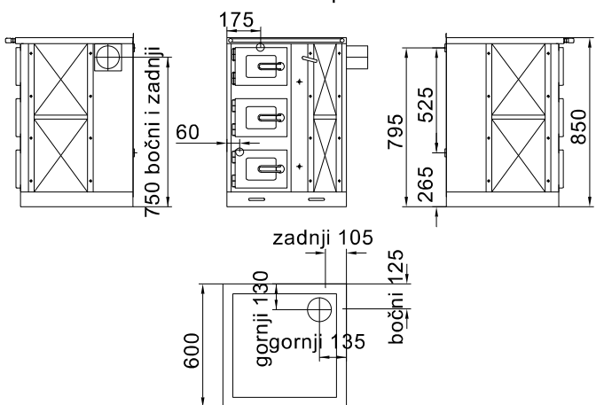
GITA CENTRAL 24kW bez pečnice
